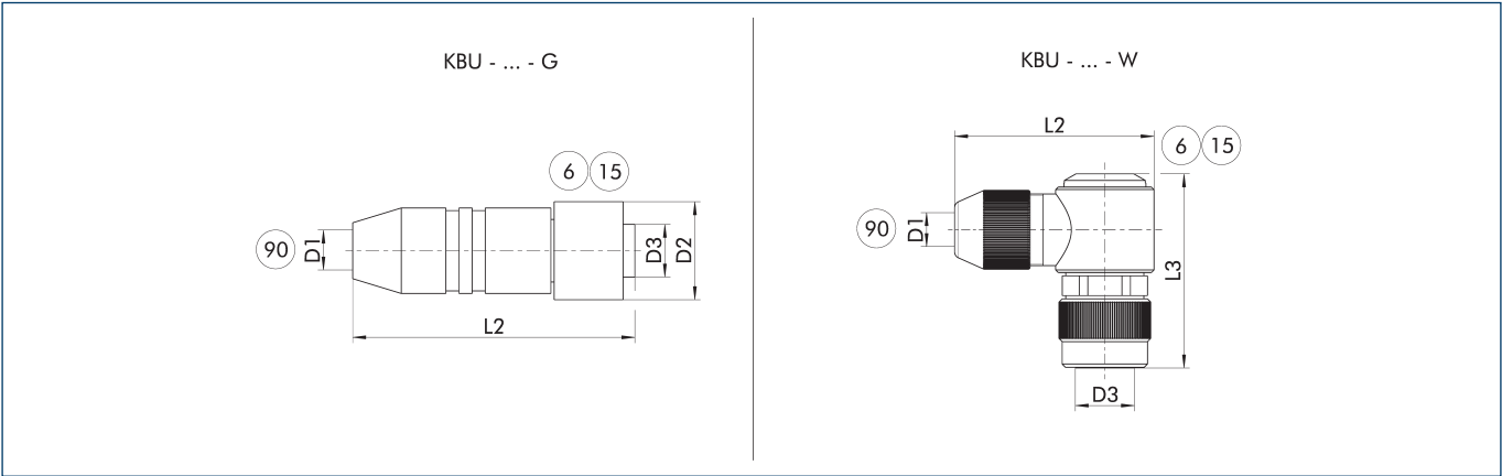
KBU - ... - G 带直插口的插座 KBU - ... - W 带角度插口的插座
