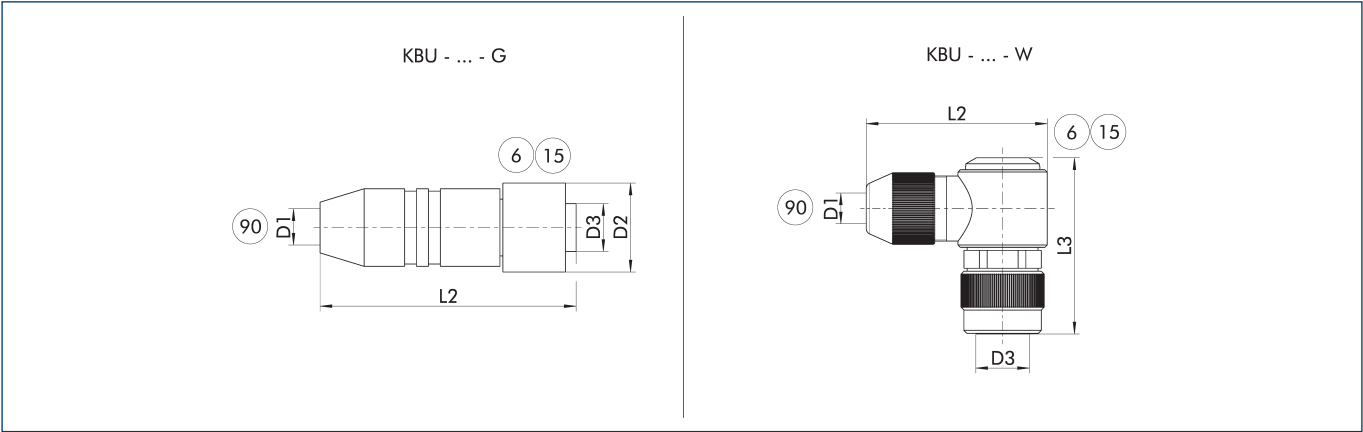
KBU - ... - G 带直插口的插座 6 连接模块侧 90 D1 - 连接电缆的最大直径 KBU - ... - W 带角度插口的插座 15 插座
