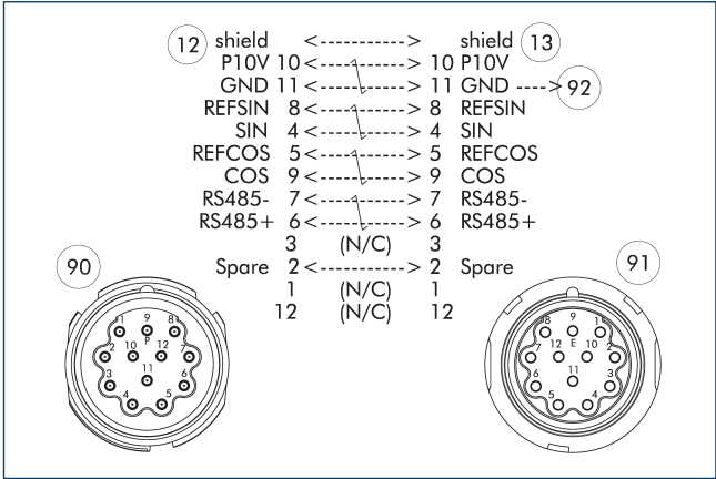
12 主侧 13 转接头侧 90 JAE 接口 91 JAE 接口 92 导引销
